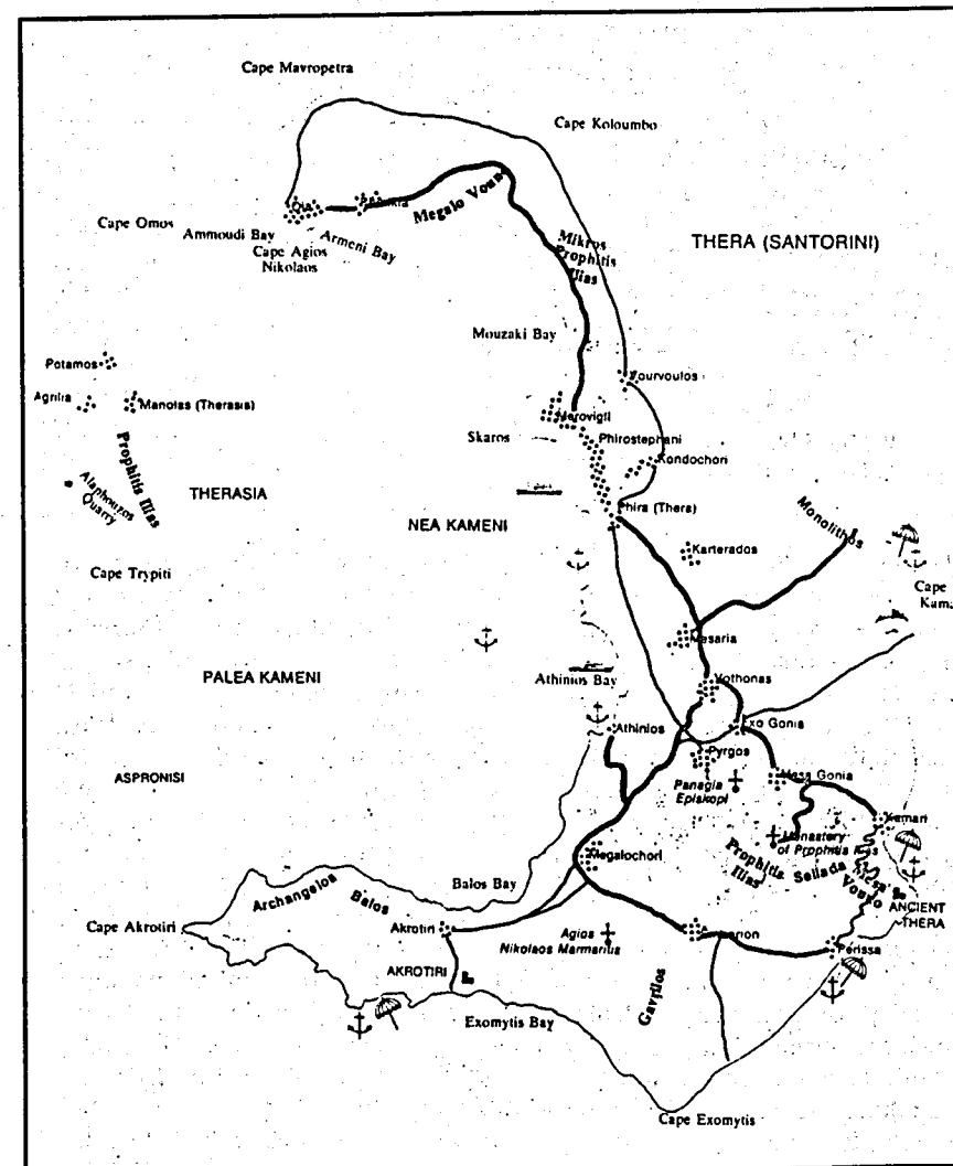
Wyspa Santorini dzisiaj. Wybuch wulkanu około roku 1600 przed Chr. zniszczył większą część wyspy pozostawiając tylko część peryferyjną. Wybuch przyczynił się do upadku kultury kretańskiej.
