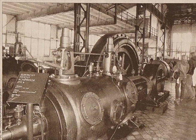
Ostrawa ma już doświadczenie z turystycznym wykorzystaniem zabytków techniki. Na zdjęciu kompresory kopalni „Michał”, tzw. muzeum ostatniego dnia - zachowu- jącego w niezmiennym stanie ostatnie chwile pracy zakładu.
